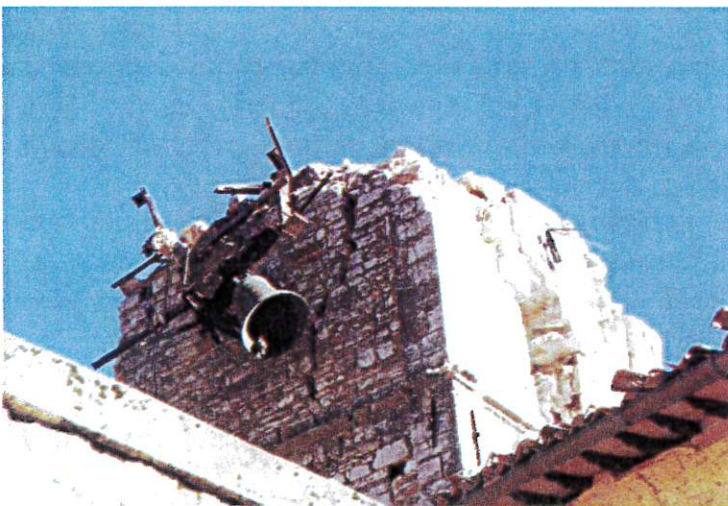
Figure 12-13 Il campanile di S. Stefano a Castelsantangelo sul Nera (MC) prima e dopo i sismi.
